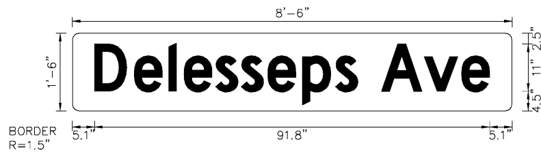
Panel Style: D3-1 #1 M.U.T.C.D.: 2009 Edition
