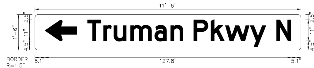
Panel Style: D3-1 #8 M.U.T.C.D.: 2009 Edition
