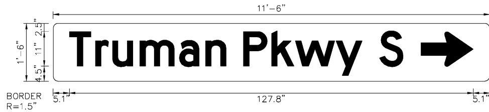
Panel Style: D3-1 #3 M.U.T.C.D.: 2009 Edition
