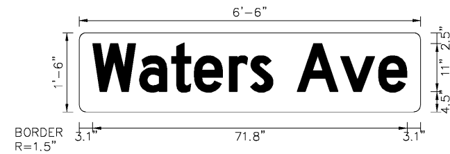
Panel Style: D3-1 #2 M.U.T.C.D.: 2009 Edition
