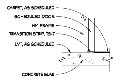
10 SILL DETAIL - CPT/LVT SCALE: 1 1/2" = 1'-0"
