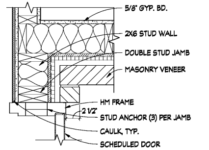
2 JAMB DETAIL SCALE: 1 1/2" = 1'-0"
