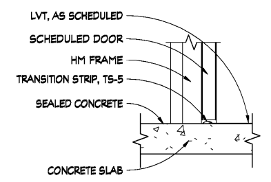
8 SILL DETAIL - SC/LVT SCALE: 1 1/2" = 1'-0"
