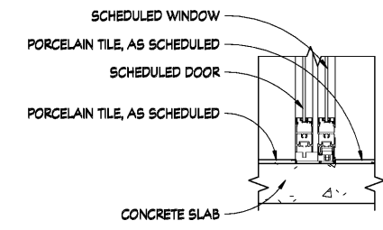
13 SILL DETAIL SCALE: 1 1/2" = 1'-0"
