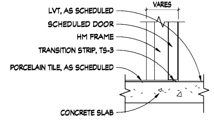
7 SILL DETAIL - PT/LVT SCALE: 1 1/2" = 1'-0"
