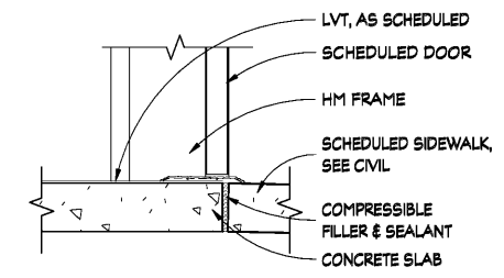
3 SILL DETAIL - SVT/EXT SCALE: 1 1/2" = 1'-0"
