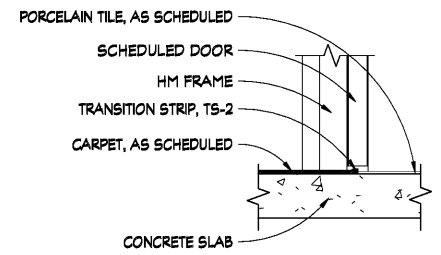
6 SILL DETAIL - CPT/PT SCALE: 1 1/2" = 1'-0"
