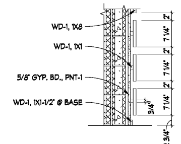
1 WALL PLANKS DETAIL A831 SCALE: 1" = 1'-0"
