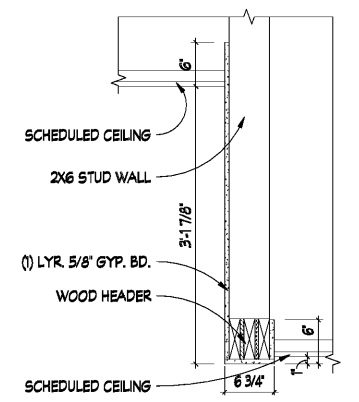
5 SOFFIT @ LOBBY/CORRIDOR A120 SCALE: 1" = 1'-0"
