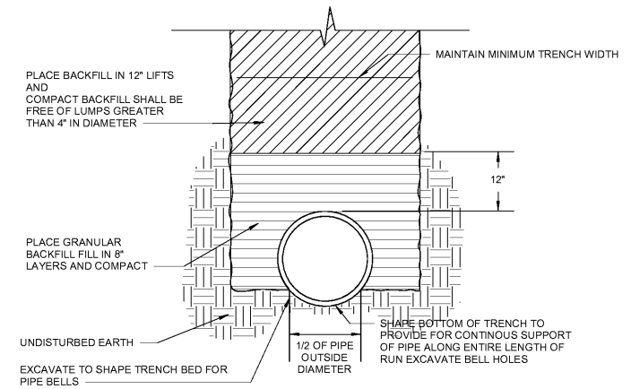
3 DETAIL - RIGID PIPE BEDDING P3.2 N.T.S.
