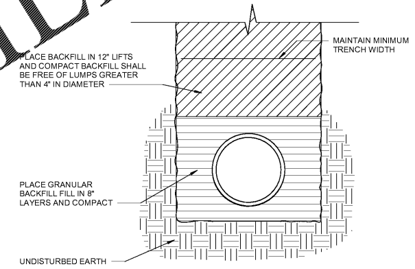
2 DETAIL - FLEXIBLE PIPE BEDDING P3.2 N.T.S.
