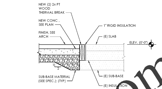
A3 Section SCALE: 3/4"=1'-0"
