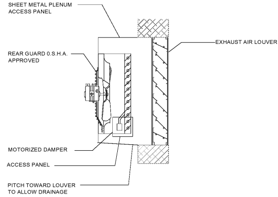
2 FAN DETAIL Scale: NTS
