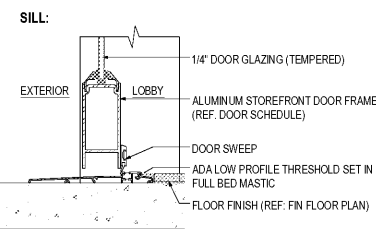
STOREFRONT 3'-1"
