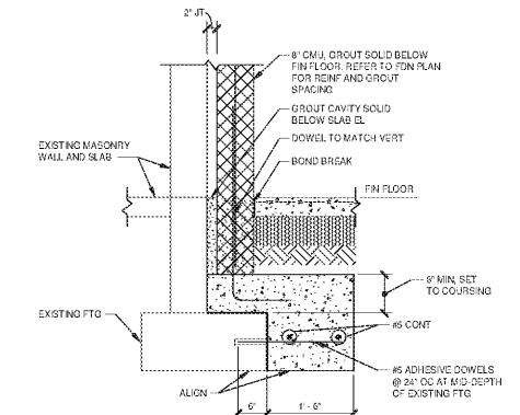
2 SECTION S1.1.1/S3.1.1 3/4\"/>
