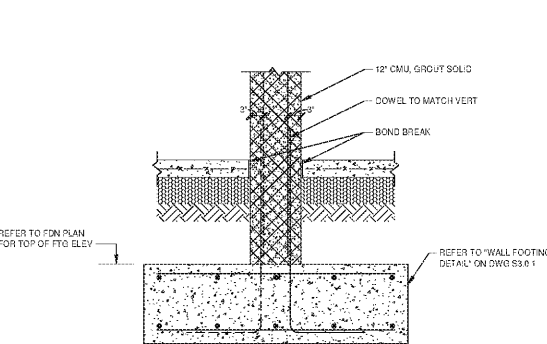
9 SECTION S1.1.1/S3.1.1 3/4\"/>
