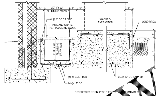
11 SECTION S1.1.1/S3.1.1 3/4\"/>
