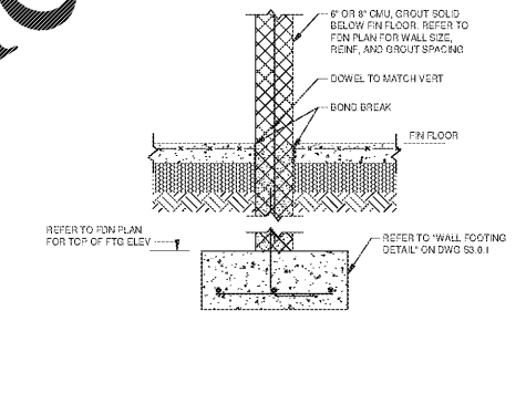
3 SECTION S1.1.1/S3.1.1 3/4\"/>
