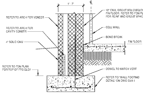
6 SECTION S1.1.1/S3.1.1 3/4\"/>
