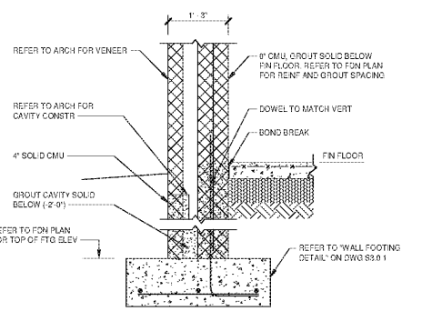
1 SECTION S1.1.1/S3.1.1 3/4\"/>
