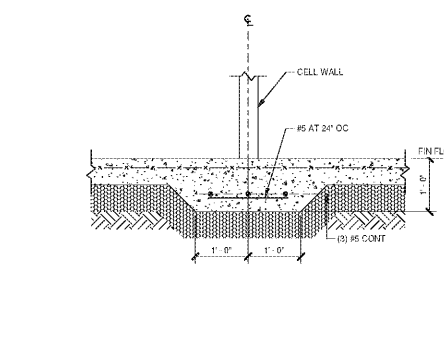
5 SECTION S1.1.1/S3.1.1 3/4\"/>
