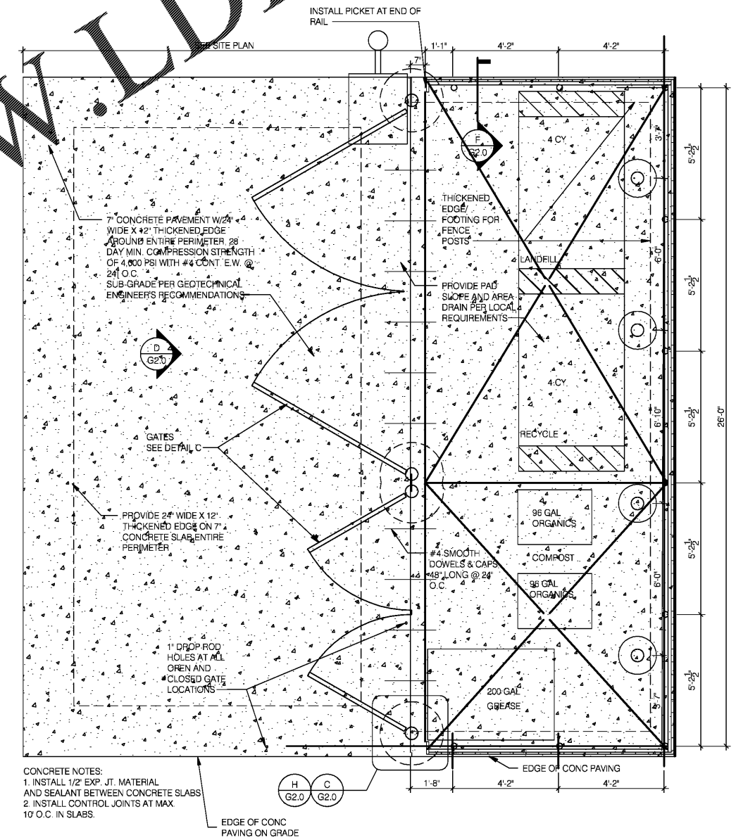
DUMPSTER PLAN N.T.S. A
