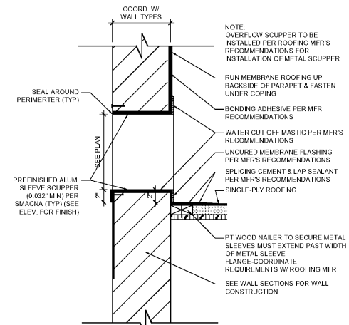
2 A-3.1 SCUPPER DETAIL SCALE: 1 1/2" = 1'-0"
