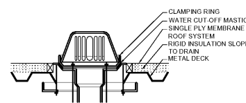
1 A-3.1 PRIMARY DRAIN SCALE: 1 1/2" = 1'-0"
