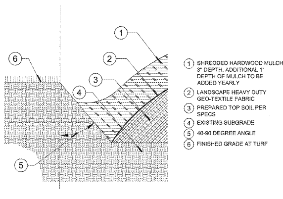
2 SHOVEL CUT BED EDGE W/ FABRIC N.T.S. DDG-GE-LA-03
