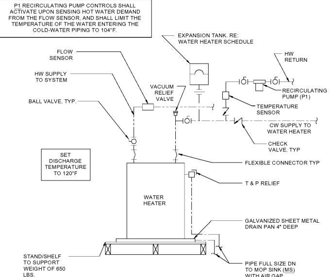
2 WATER HEATER N.T.S.
