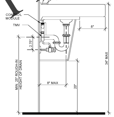
4 LAV SHROUD N.T.S.
