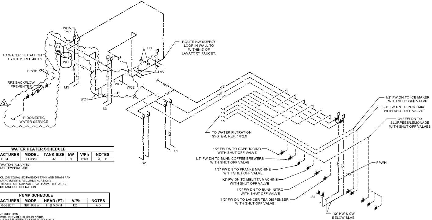
2 WATER RISER N.T.S.
