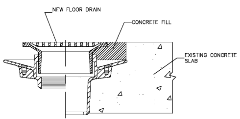
2 FLOOR DRAIN DETAIL N.T.S.
