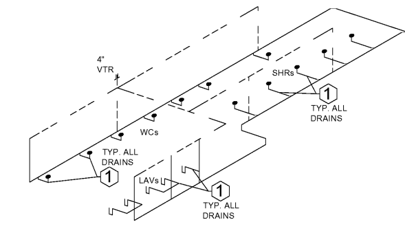
3 SEWER ISOMETRIC PLAN N.T.S.
