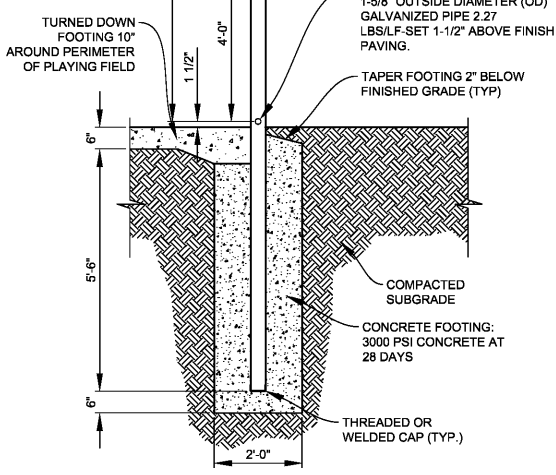
24' HIGH BACKSTOP SCALE: N.T.S.
