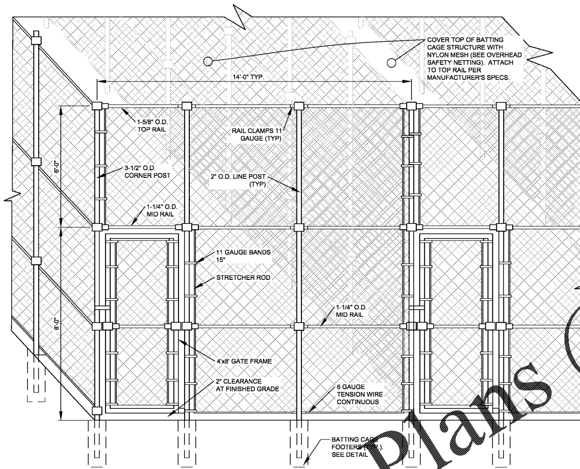
BATTING CAGE SCALE: N.T.S.
