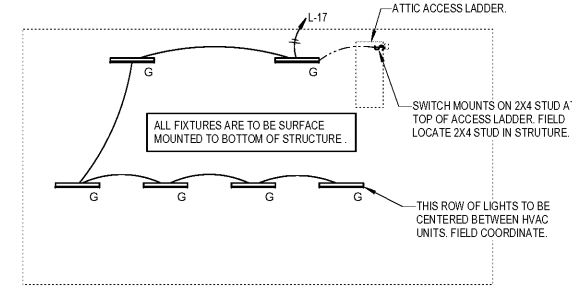
2 Attic Floor SCALE: 1/8" = 1'-0"
