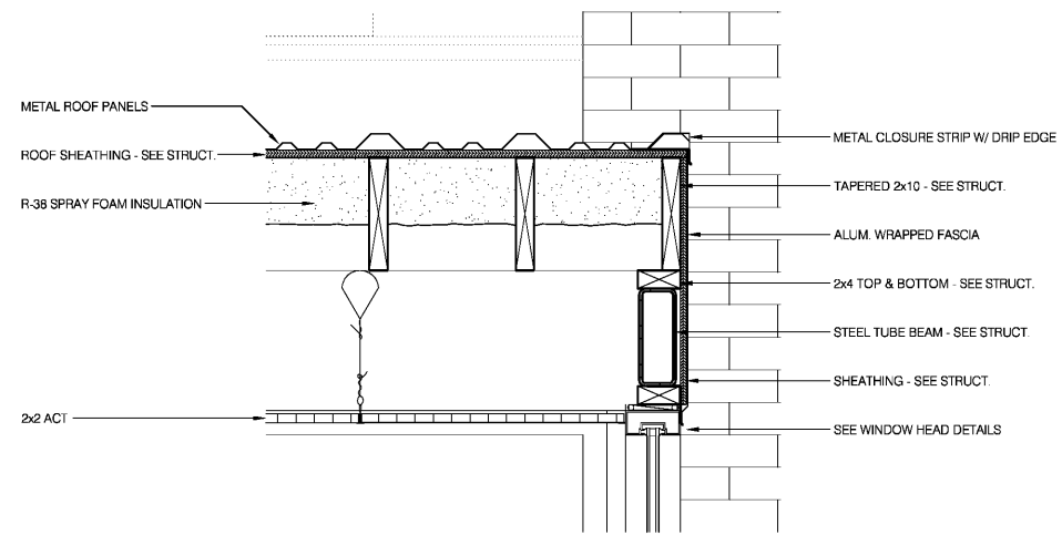
1 A408 1 1/2" = 1'-0"
