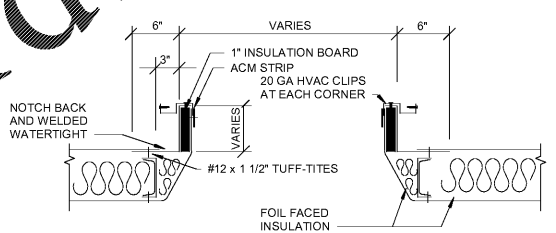
3 ROOF CURB DETAIL M2 N.T.S.
