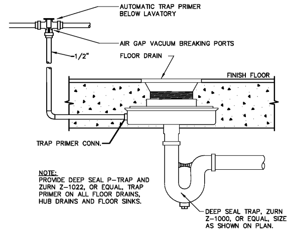
TRAP PRIMER DETAIL
