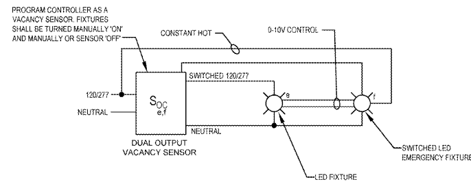
BREAK ROOM CONTROL SCHEME N.T.S.
