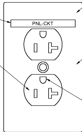
C1 RECEPTACLE DETAIL (TYP.)
