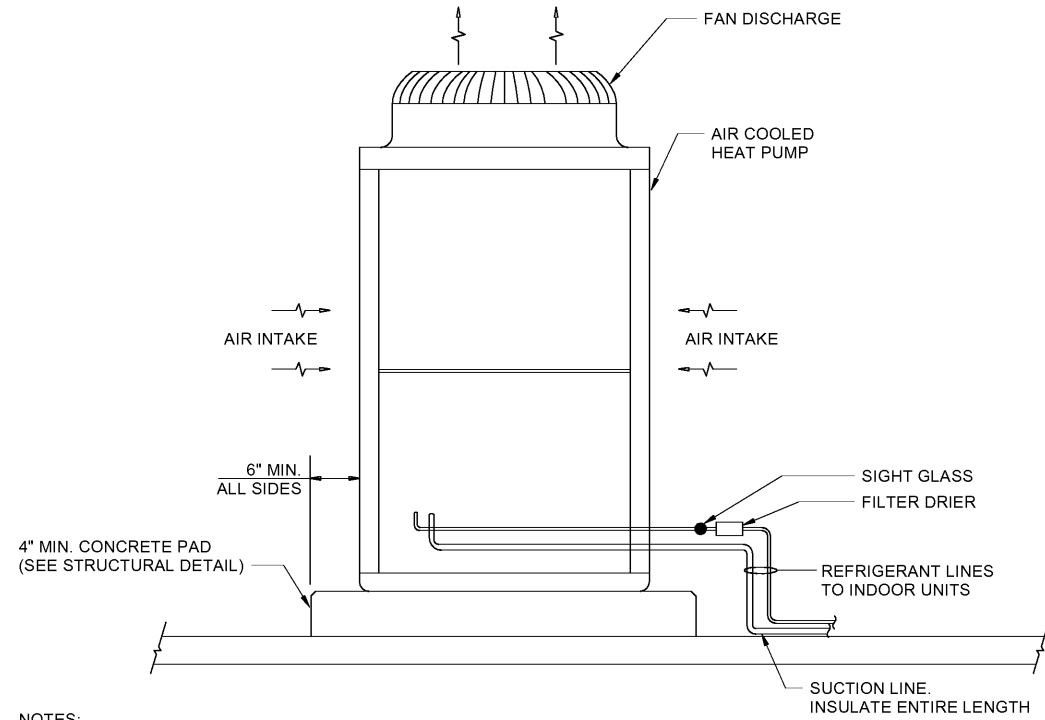
C1 VRF HEAT PUMP DETAIL SCALE: N.T.S.
