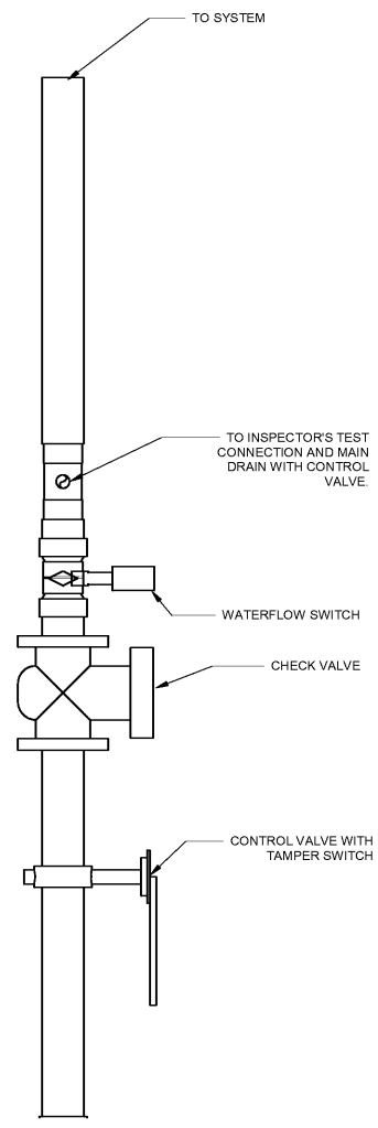
A4 TYPICAL WET-PIPE RISER ASSEMBLY DETAIL SCALE: N.T.S.
