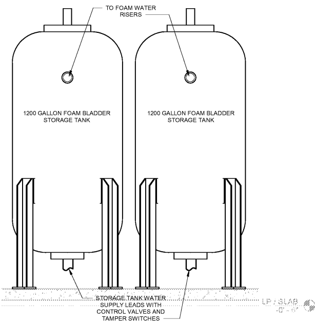
C1 FOAM STORAGE TANKS DETAIL SCALE: N.T.S.
