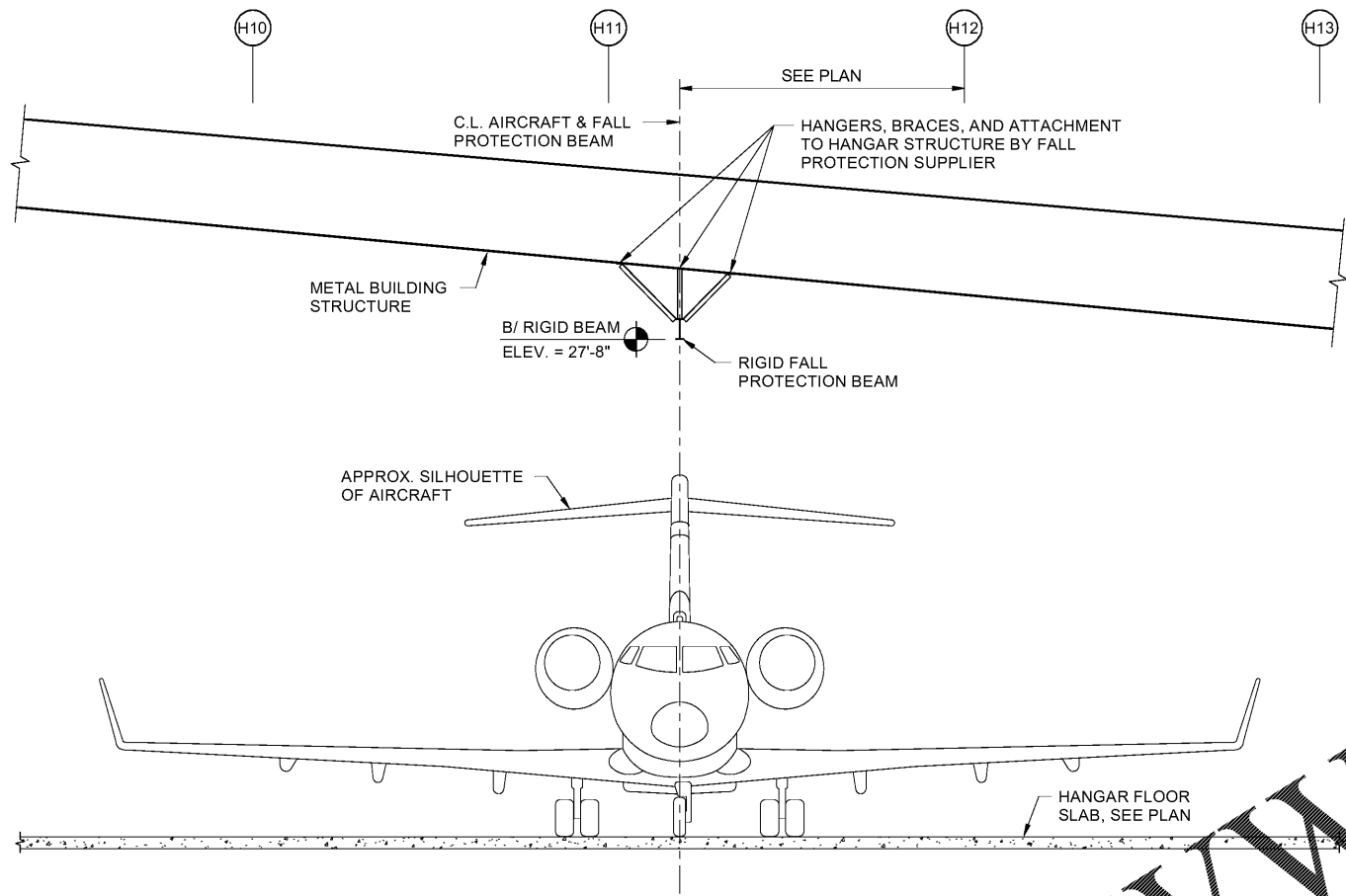
B1 FALL PROTECTION SECTION SCALE: N.T.S.
