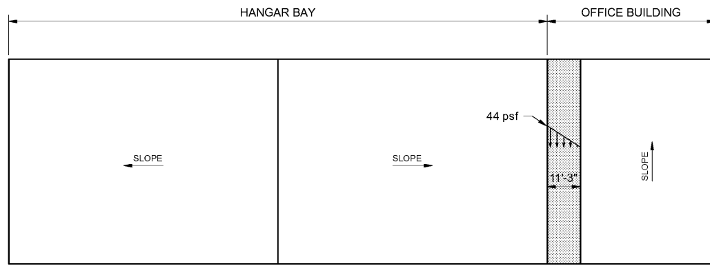
C1 SNOW DRIFT DIAGRAM SCALE: N.T.S.
