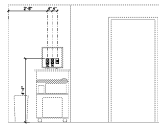
3 LOUNGE SCALE: 1/2" = 1'-0"
