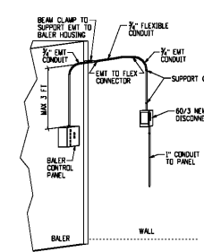
21 BALER CONNECTION ELEVATION SCALE: N.T.S.
