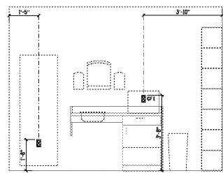
1 LOUNGE SCALE: 1/2" = 1'-0"
