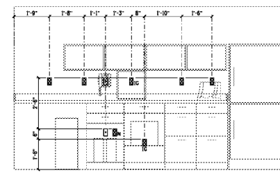
11 CASH ROOM SCALE: 1/2" = 1'-0"
