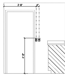
10 CASH ROOM SCALE: 1/2" = 1'-0"
