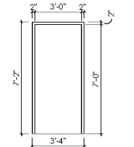
DOOR FRAME SCALE: 1/4" = 1'-0"
