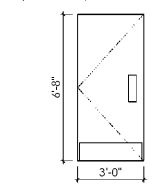
DOOR SCALE: 1/4" = 1'-0"
