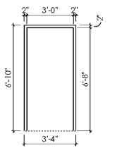
DOOR FRAME SCALE: 1/4" = 1'-0"
