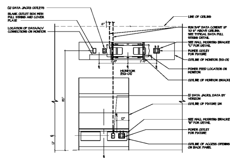
1 POWER DIAGRAM FOR EQ-O & DR N.T.S.
