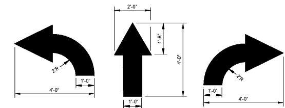
DIRECTIONAL ARROW DETAIL N.T.S.
