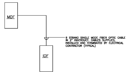
MDF FIBER OPTIC CABLE RISER DIAGRAM N.T.S.
