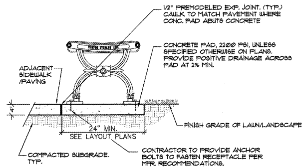
2 BENCHES SCALE: NTS
