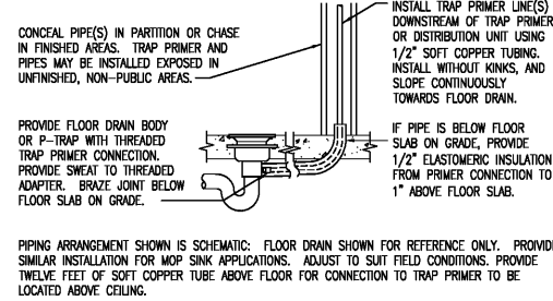
3 TRAP PRIMER INSTALLATION NO SCALE
