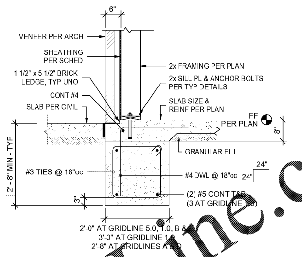
C FOUNDATION SECTION S-7 N.T.S.
