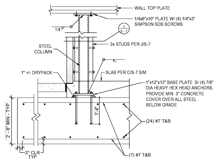
F FOUNDATION SECTION S-7 N.T.S.
