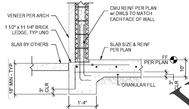
B FOUNDATION SECTION S-7 N.T.S.
