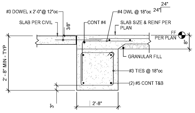
G FOUNDATION SECTION S-7 N.T.S.
