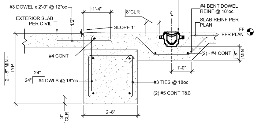
A FOUNDATION SECTION S-7 N.T.S.
