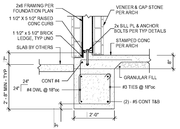
D FOUNDATION SECTION S-7 N.T.S.
