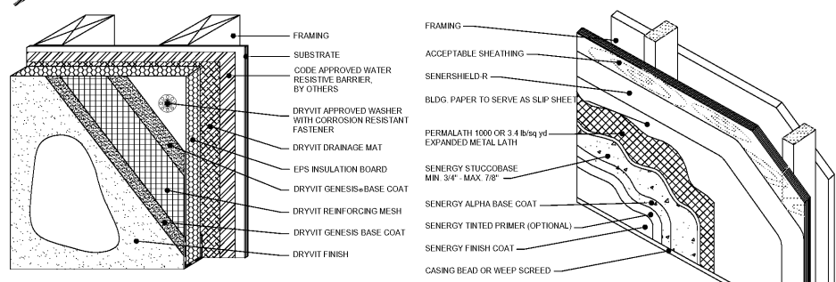
3A TYP. EIFS DETAIL
