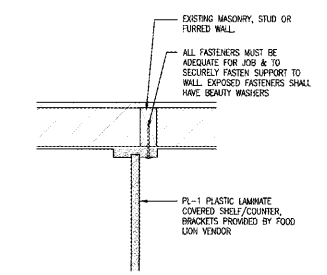
18 SECTION A4.06 SCALE: 1 1/2" = 1'-0"
