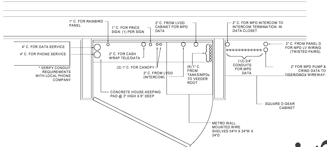
6 TELEPHONE BACKBOARD DETAIL N.T.S.
