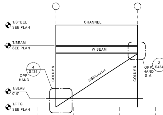
1 BRACED FRAME ELEVATION N.T.S.
