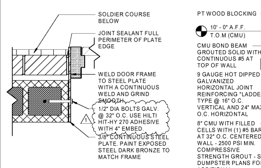
11 DOOR JAMB 1 1/2" = 1'-0"
