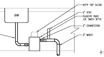
7 PLASTER TRAP PIPING SCALE: NO SCALE
