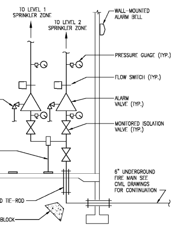
8 SPRINKLER ZONE RISER SCALE: NONE
