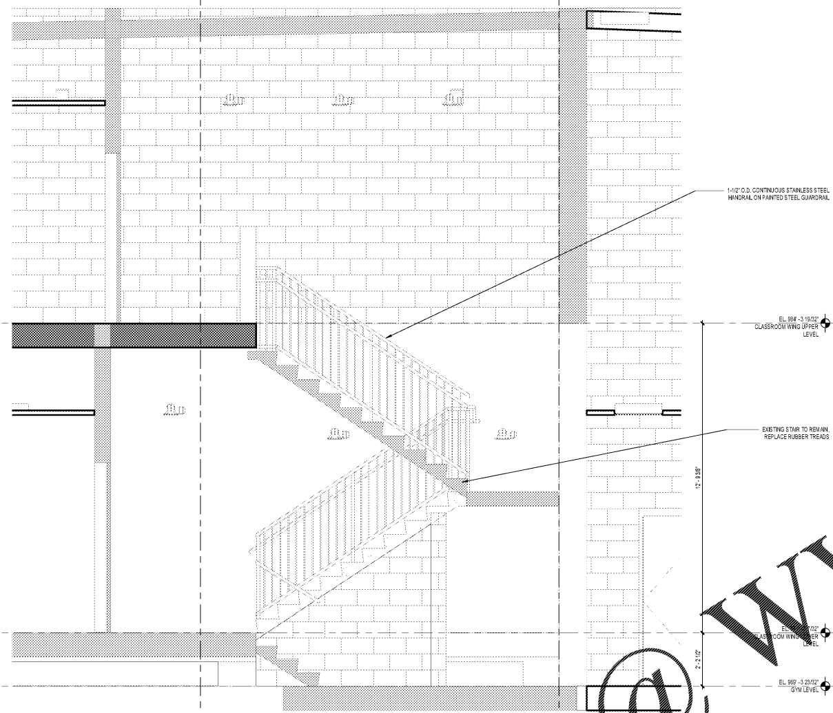
6 SECTION - STAIR 1121 A7.13 SCALE: 1/2" = 1'-0"
