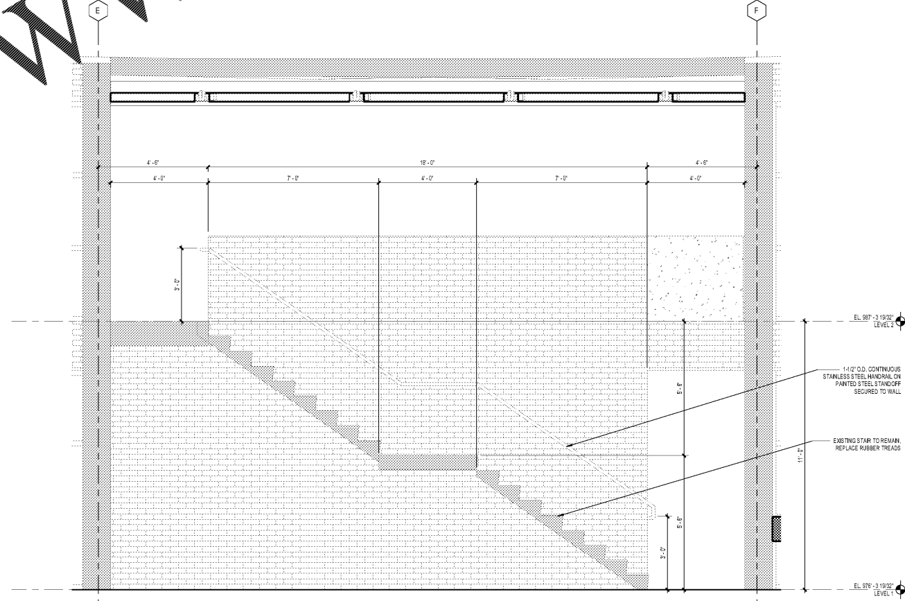
1 SECTION - STAIR 905 SCALE: 1/2" = 1'-0"
