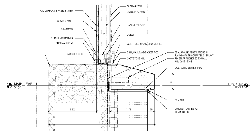
6 SECTION DTL - POLYCARB SCALE: 3" = 1'-0"
