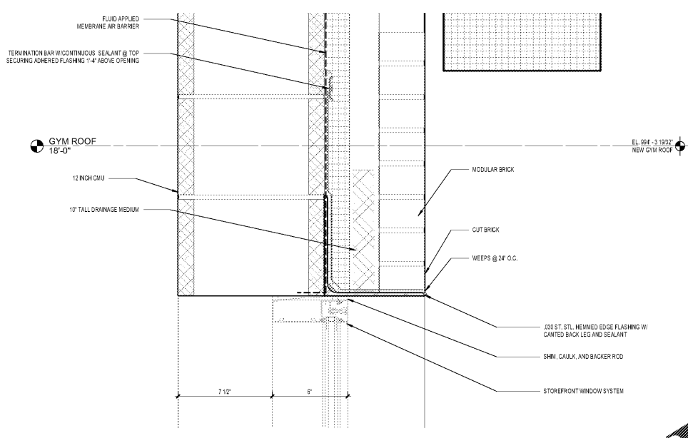
8 SECTION DTL - STOREFRONT HEAD DTL SCALE: 3" = 1'-0"
