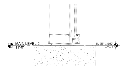
3 A5.01 ENTRY VESTIBULE - EXT. STOREFRONT SILL DETAIL SCALE: 3" = 1'-0"
