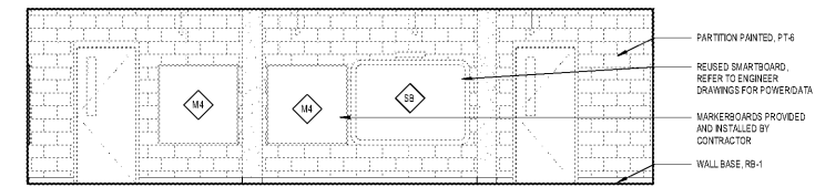
8 ELEVATION - SCI / TECH C A4.26 SCALE: 1/4" = 1'-0"
