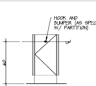
1/C - DOOR ELEVATION
