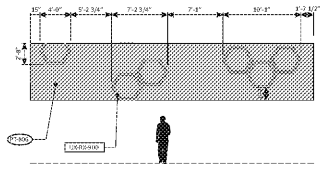
F - INTERIOR ELEVATION SCALE: 1/8" = 1'-0"
