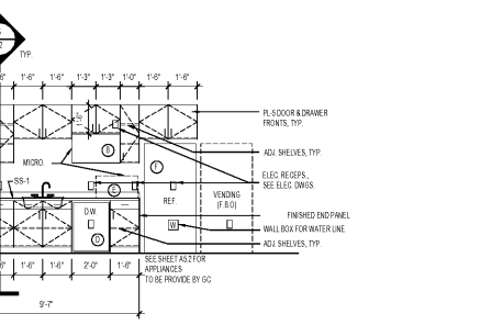
ELEV. 11
