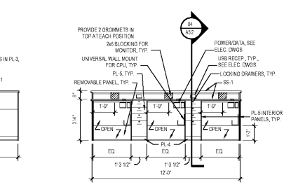
ELEVATION 17
