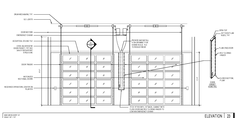
ELEVATION 23
