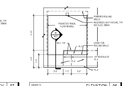
ELEV. 07
