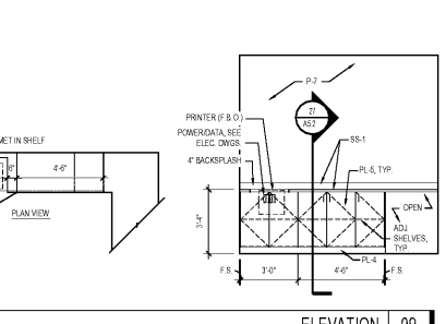
ELEVATION 09
