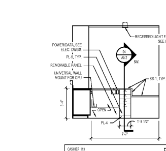
ELEV. 11
