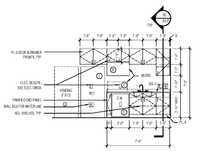
ELEVATION 10
