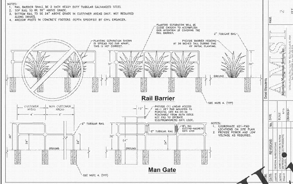
2 Rail Barrier N.T.S.
