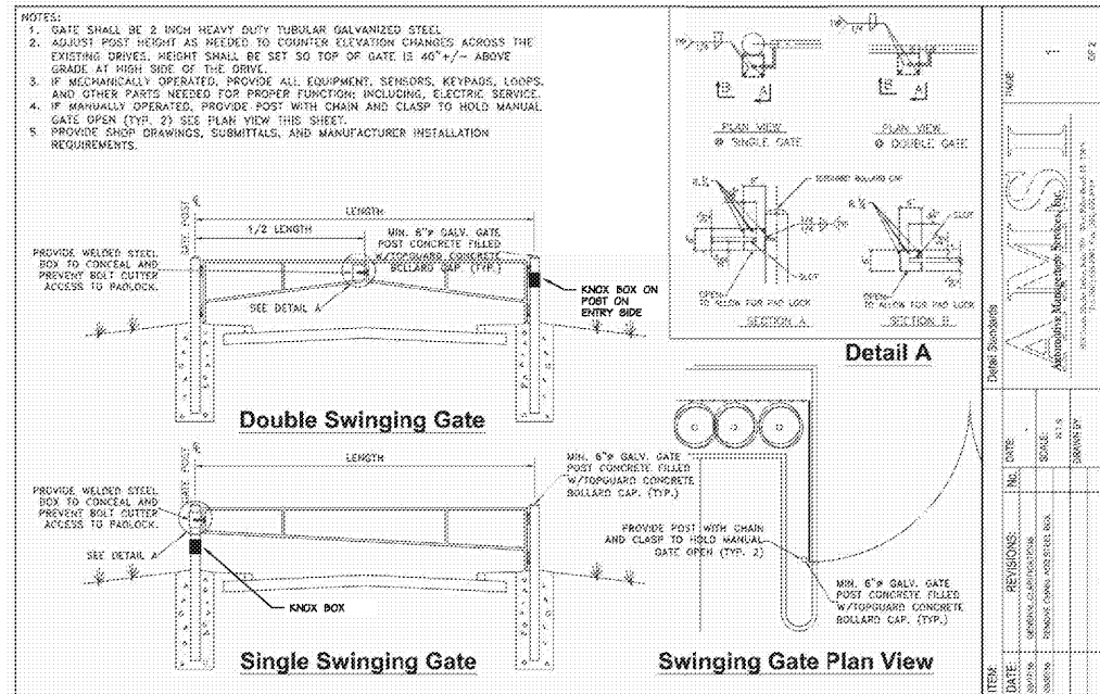
1 Swing Gates N.T.S.
