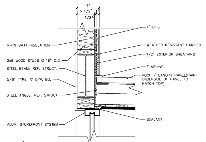
5 DETAIL SCALE: 1 1/2" = 1'-0"
