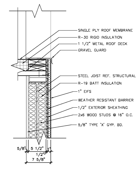
1 DETAIL SCALE: 1 1/2" = 1'-0"
