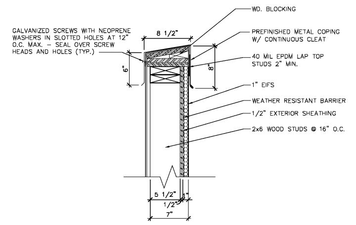
2 COPING DETAIL SCALE: 1 1/2" = 1'-0"
