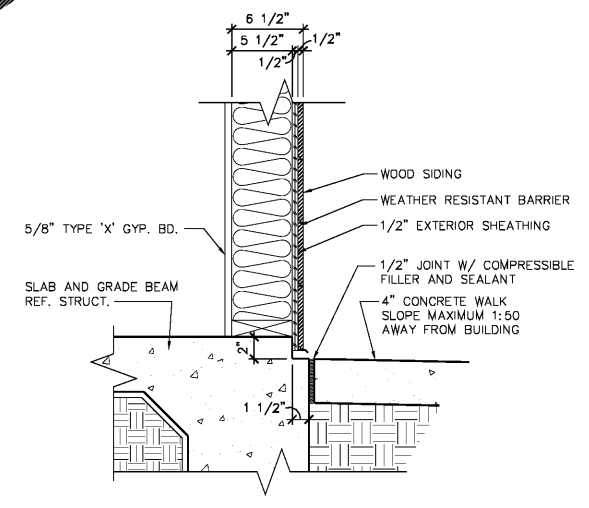
8 DETAIL SCALE: 1 1/2" = 1'-0"
