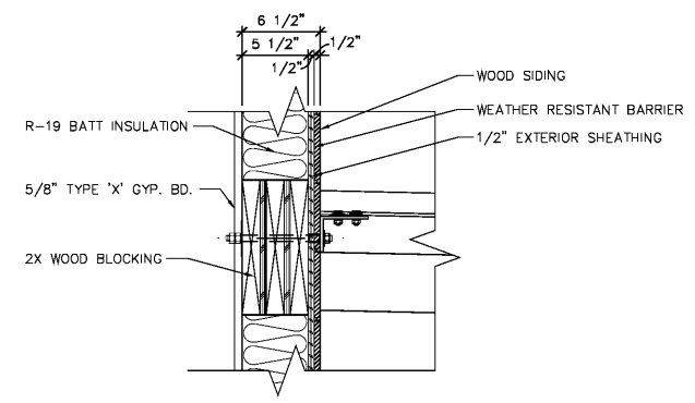
3 DETAIL SCALE: 1 1/2" = 1'-0"
